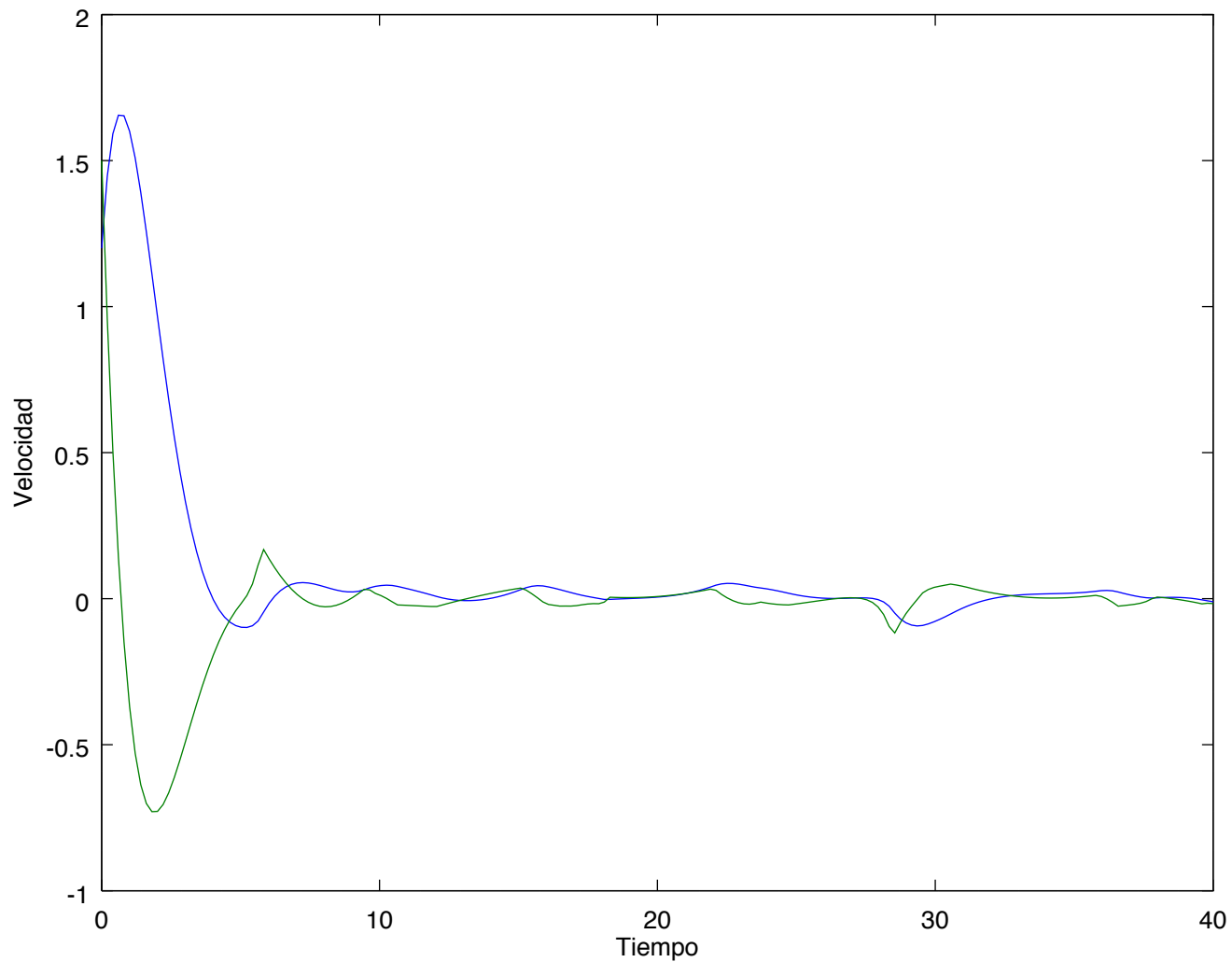
Movimiento browniano con amortiguamiento
